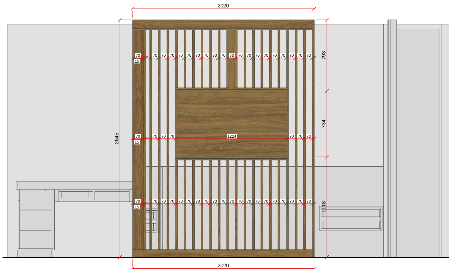
DIVISÓRIA RIPADA - ESC. 1:25
