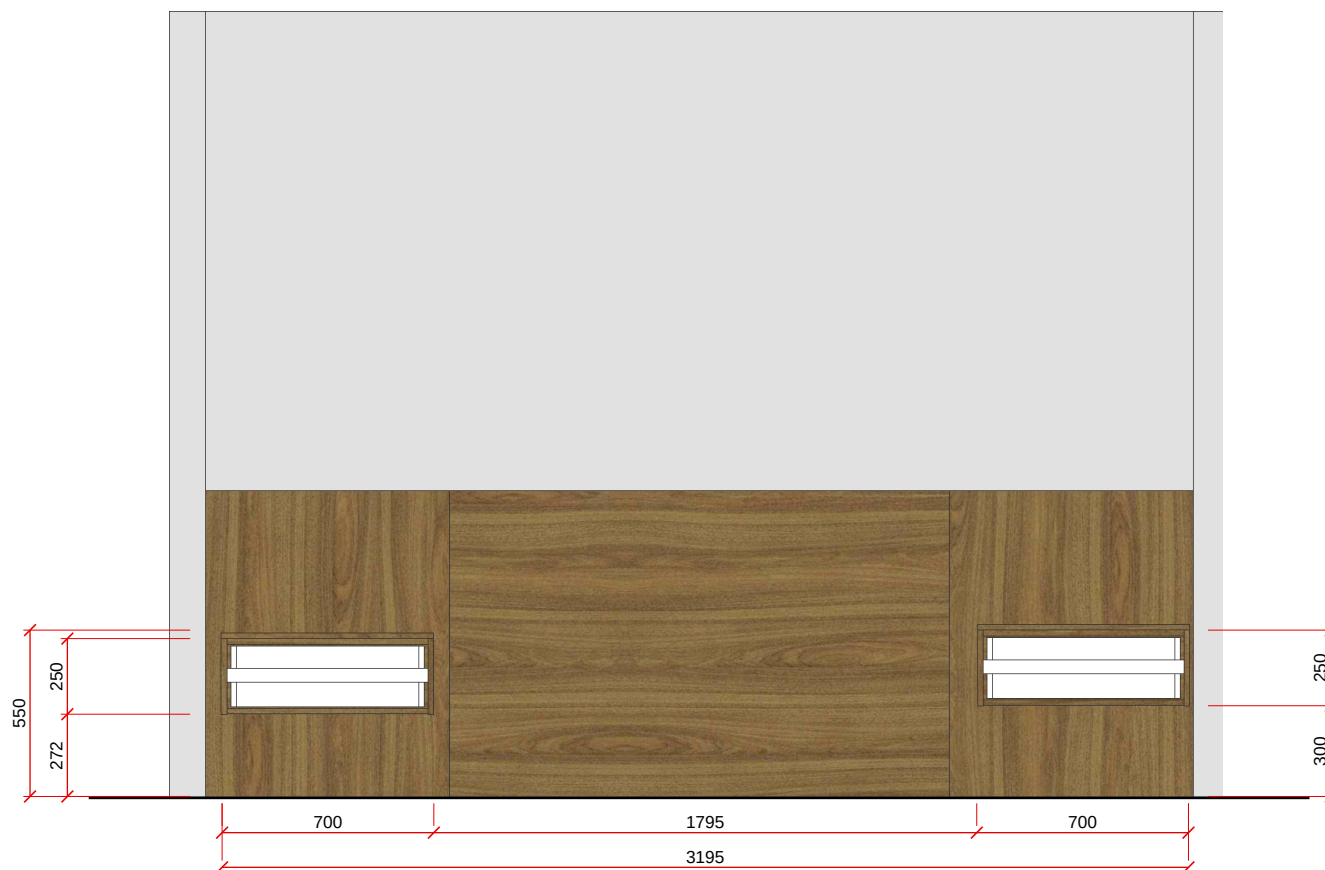
VISTA D - ESC. 1:25
